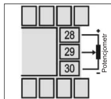
Rys. 7 podłączenie potencjometru
