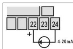
Rys. 5 podłączenie 4-20mA
