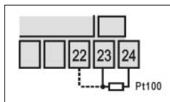
Rys. 4 Okablowanie Pt100 z zastosowaniem trzech przewodów
