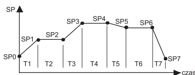
Rys. 8 – Przykład programu rampingu i wygrzewania
