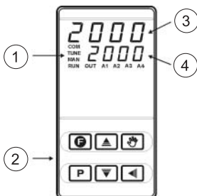
Rysunek 1 – Przedni panel
