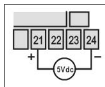
Rys. 6 podłączenie 5 VDC
