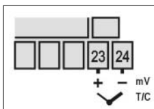
Rys. 3 Termopara i 0-50mV
