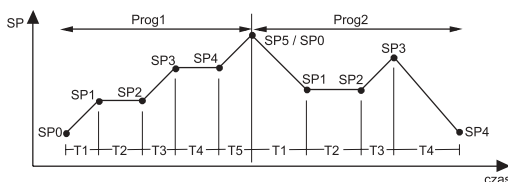
Rys. 10 – Przykład połączenia programów 1 i 2
