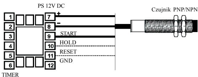
Rysunek 2 - Podłączenie czujnika typu PNP/NPN
